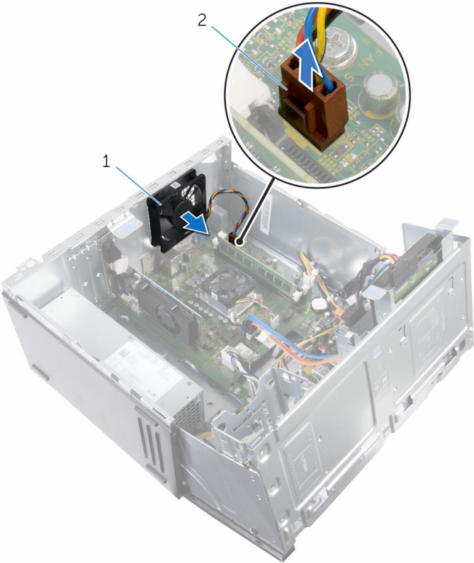
1 chassis fan
