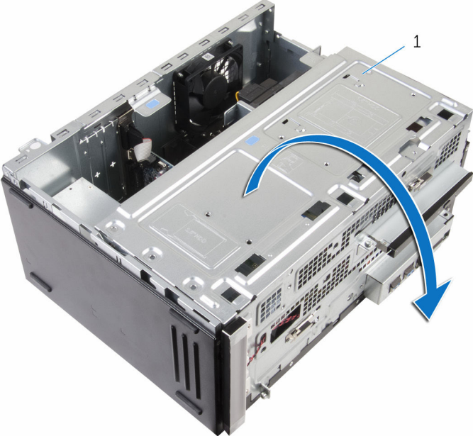
1 side-chassis
